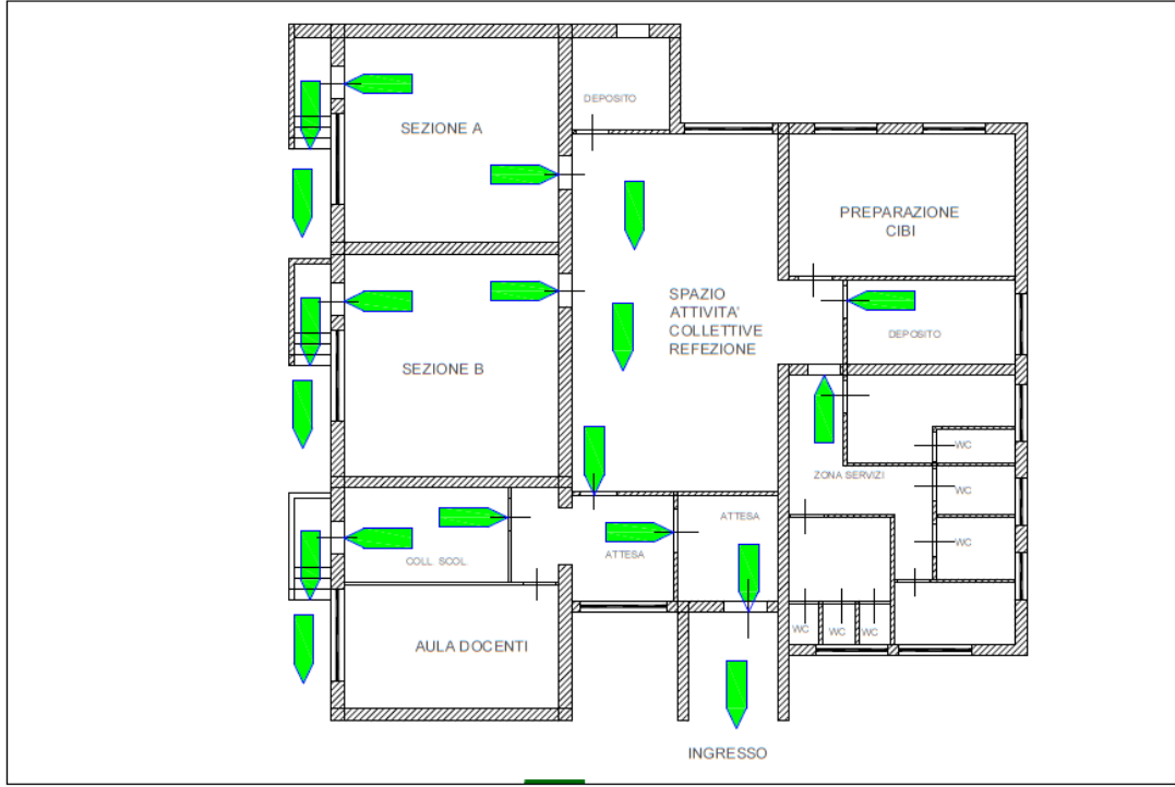
S.SOSTI- SCUOLA INFANZIA- PIANO TERRA-PERCORSI-EVACUAZIONE
