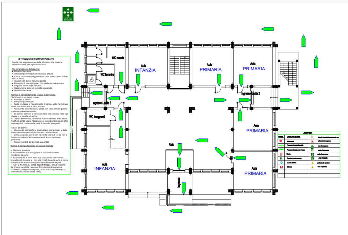
S.SOSTI-INFANZIA-PRIMARIA- PIANO TERRA-PIANO DI EVACUAZIONE
